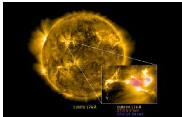
Die Instrumente EUVI und STIX wurden Zeuge einer Sonneneruption, die am 2. März 2022 ausbrach.
